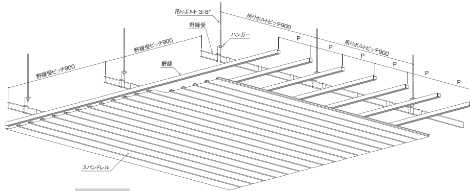
天井部納まり
