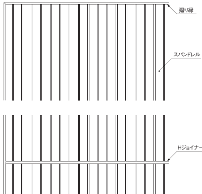
《施工部位の天井下地材と下地間隔》
