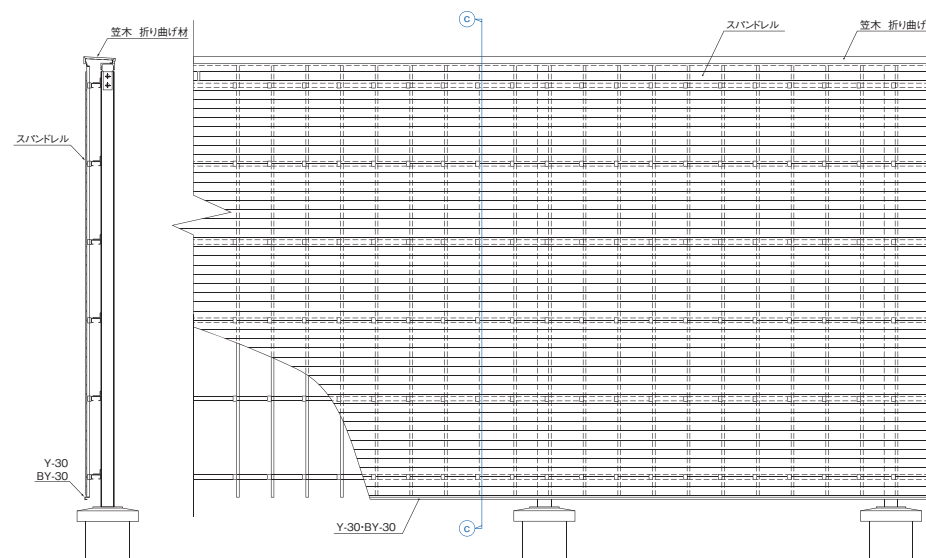
c-c 断面図
