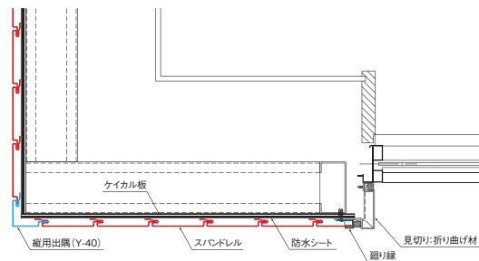
b 断面図
