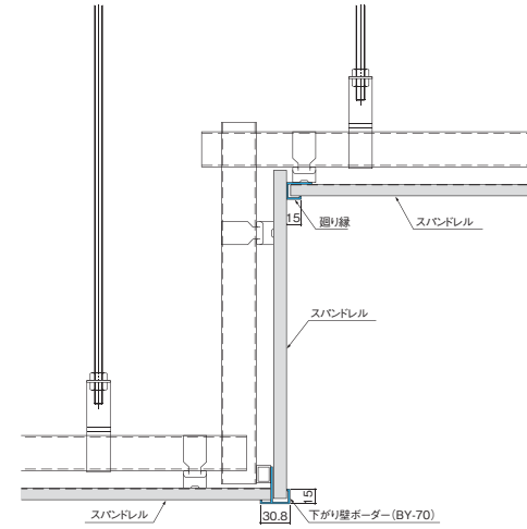
下がり壁納まり
