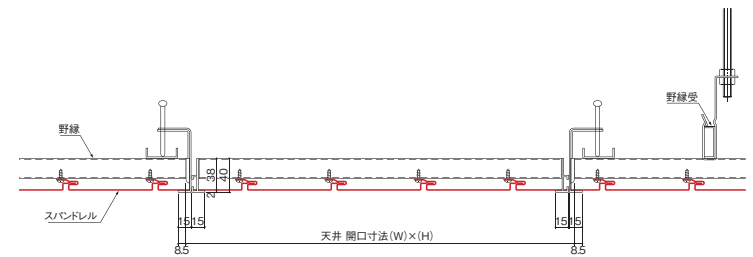
天井点検口納まり図
