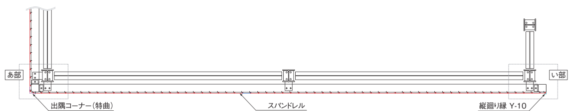
B断面
