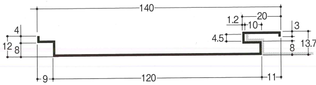
AS120 (目地無しタイプ) 板厚 t=1.2\text{mm} /働き幅: 120mm
