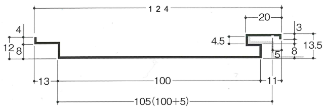
AS101 板厚t=1.0mm/働き幅：100mm
