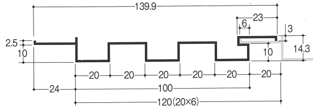
AS110 板厚 t=1.1\text{mm} /働き幅: 120mm
