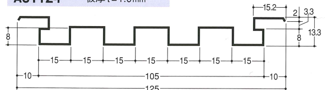
AS112-F 板厚t=1.0mm
