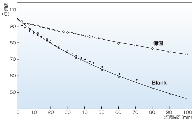
保温効果例 (外気温度 \theta_o=1^{\circ}\text{C} )
