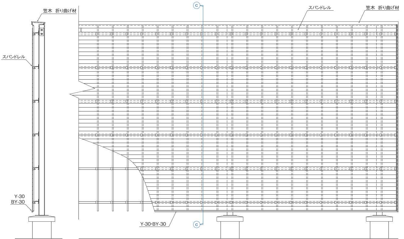
C-C 断面図
